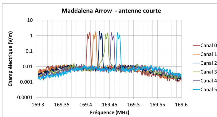
Figure 6 : signatures fréquentielles des signaux émis selon le canal choisi pour le module Maddalena Arrow avec l'antenne courte
