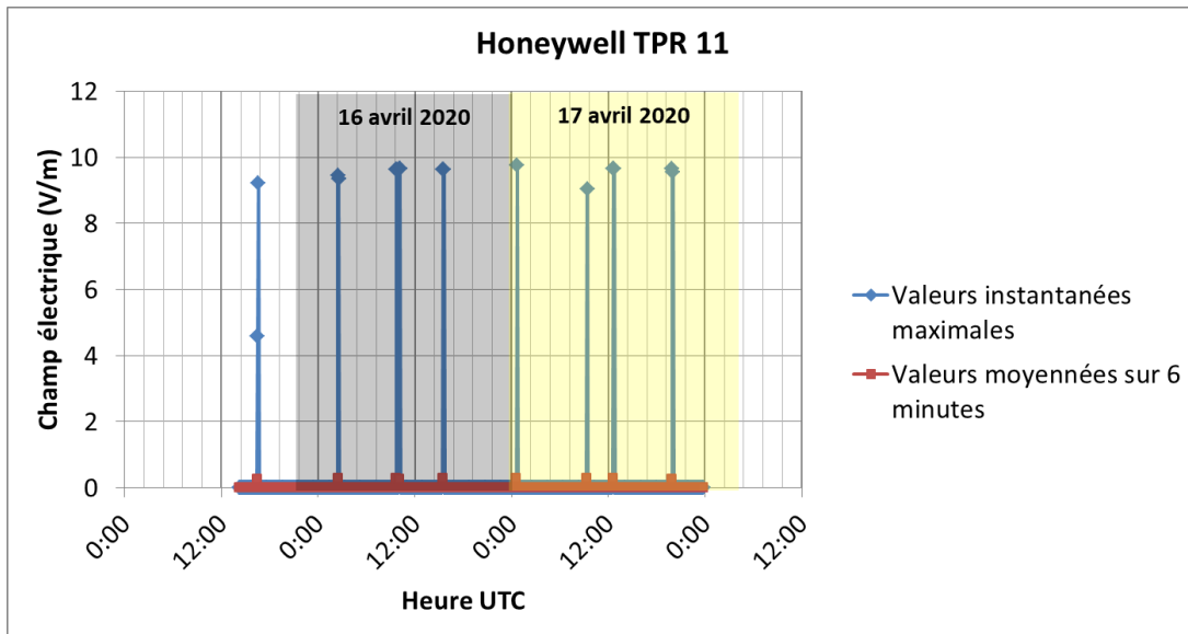
Figure 12 : relevés des niveaux de champ instantané maximal et moyenné sur 6 minutes à 25 cm des compteurs sur une durée d'au moins 2 jours.
