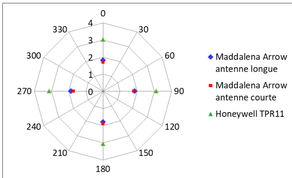
Figure 8 : niveaux de champ électrique crête mesurés dans les 4 directions principales autour des modules dans un plan horizontal
