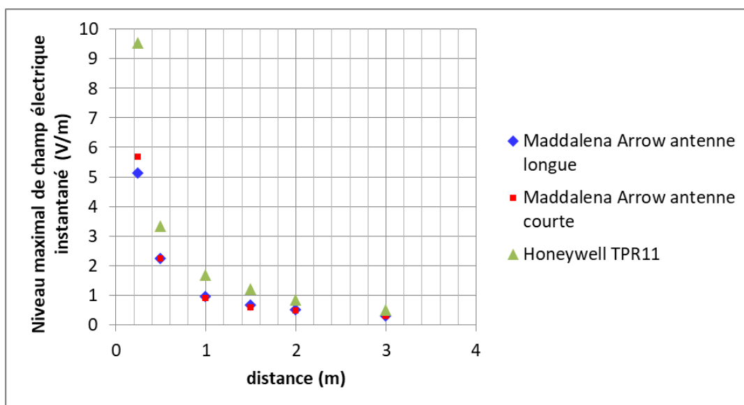
Figure 9 : décroissance des niveaux de champ électrique crête émis par les modules en fonction de la distance
