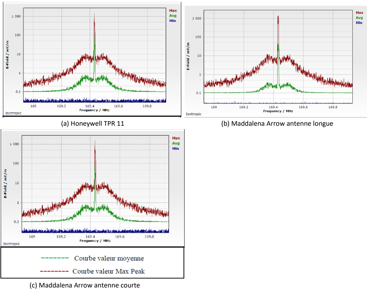
Figure 11 : analyse spectrale des émissions des modules testés relevés lors des essais COFRAC
